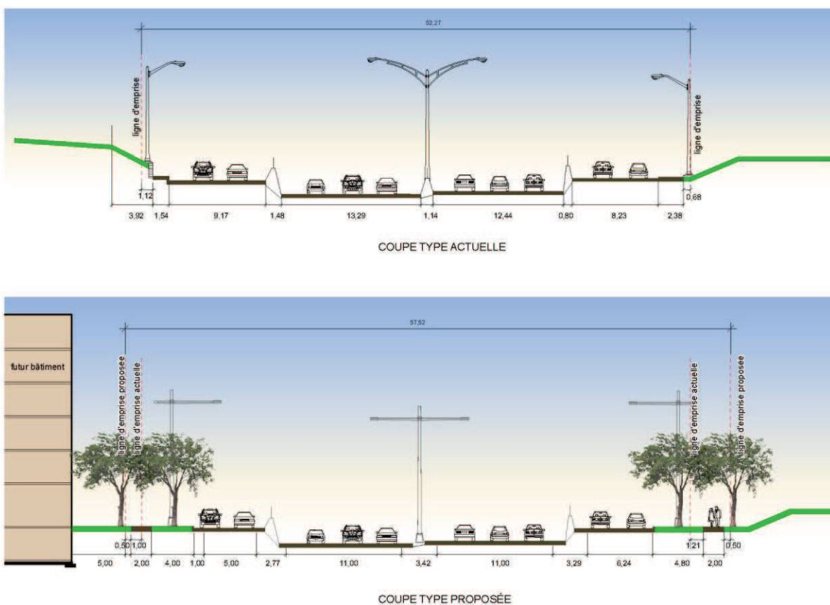
Figure 44 : Coupe type de l'axe Robert-Bourassa
