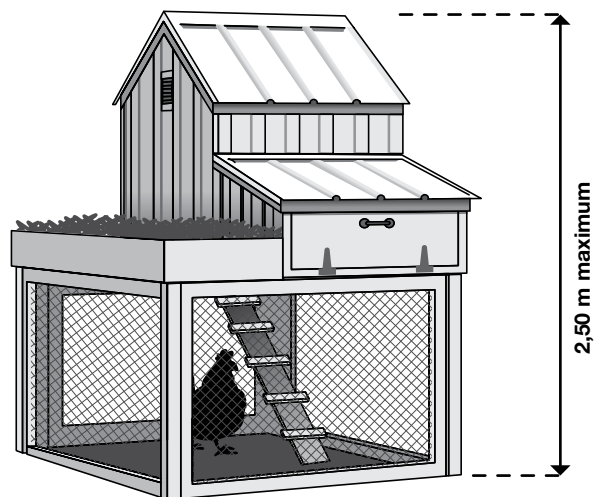
CROQUIS 1 – ENCLOS FERMÉ SOUS LE POULAILLER
