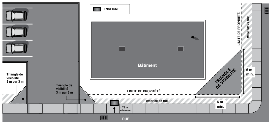
CROQUIS 2 – LOCALISATION
