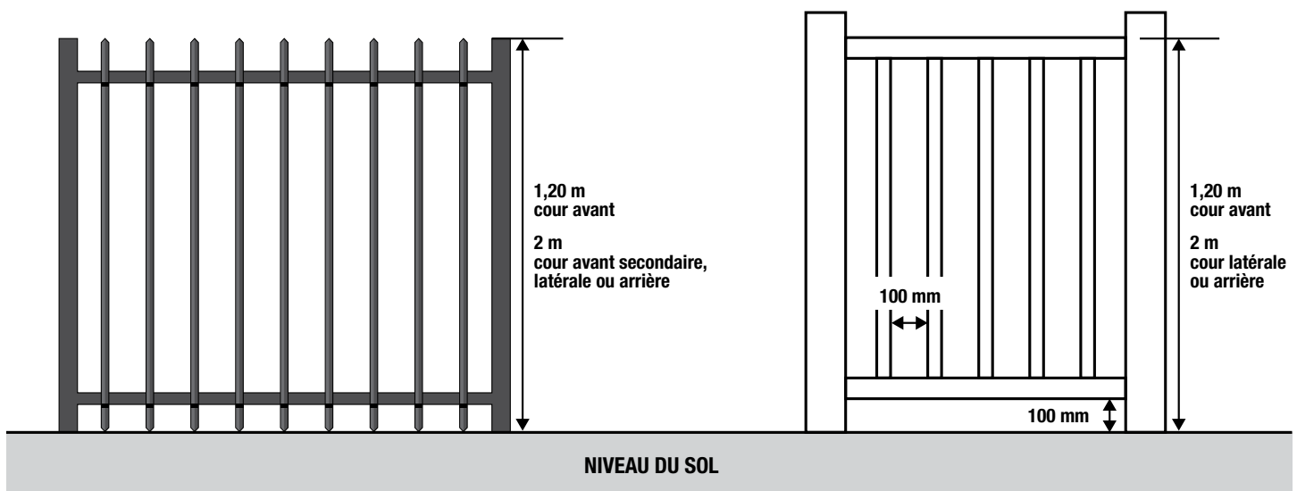
CROQUIS 3 – CLÔTURE
