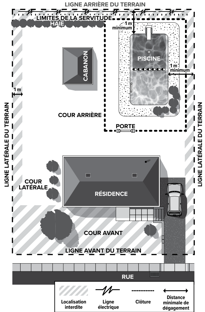
CROQUIS 1 – DISTANCES MINIMALES DE DÉGAGEMENT
